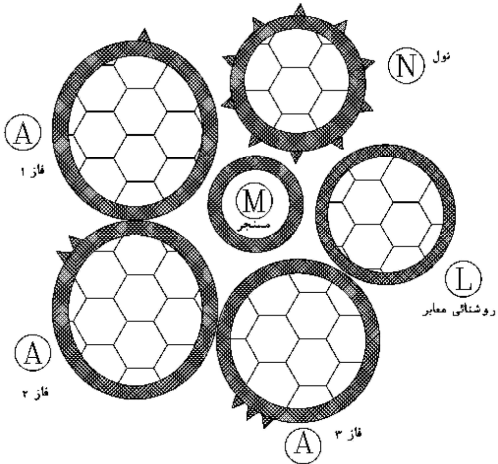
شکل شماره (۱) - برش مقطع کابل خودنگهدار شش سیمه و علامت‌های مشخصه رشته‌ها
