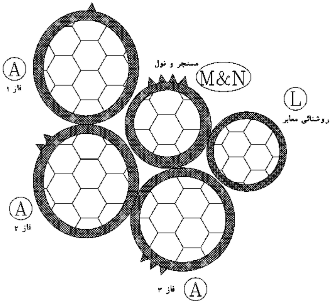
شکل شماره (۱) - برش مقطع کابل خودنگهدار پنج سیمه و علامت‌های مشخصه رشته‌ها
